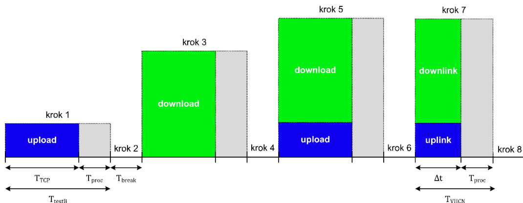
Obř. 6: Doporučená podoba procesu měření souboru datových parametrů tvořící kritéria výkonnosti VHCN dle aktuálně platných Pokynů BEREC VHCN a standardu Y.1540
