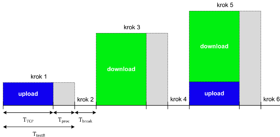
Obr. 1: Doporučená podoba procesu měření TCP propustnosti
