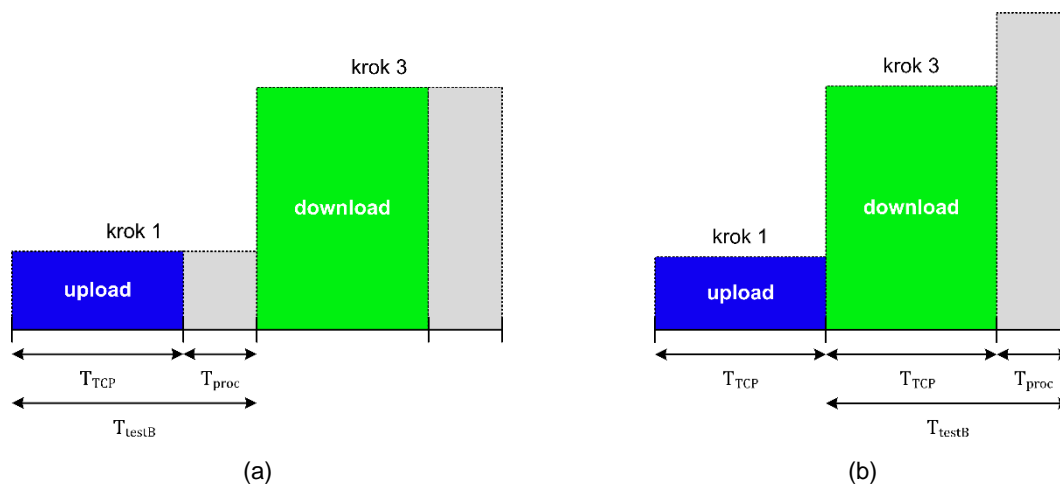
Obr. 2: Varianty minimální přípustné podoby procesu měření TCP propustnosti: (a) proces zpracování každého jednosměrného testu zvlášť, (b) proces zpracování všech jednosměrných testů na závěr samotného procesu měření
