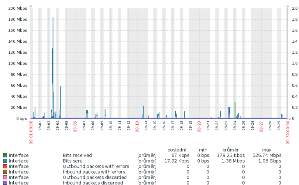
Obr. 6: Příklad průběhů rychlostí ve směru přicházejícího ( Bits received ) a odcházejícího ( Bits sent ) síťového provozu do peeringového uzlu NIX.CZ příslušného rozhraní hraničního routeru systému MSEK, DeP 1
