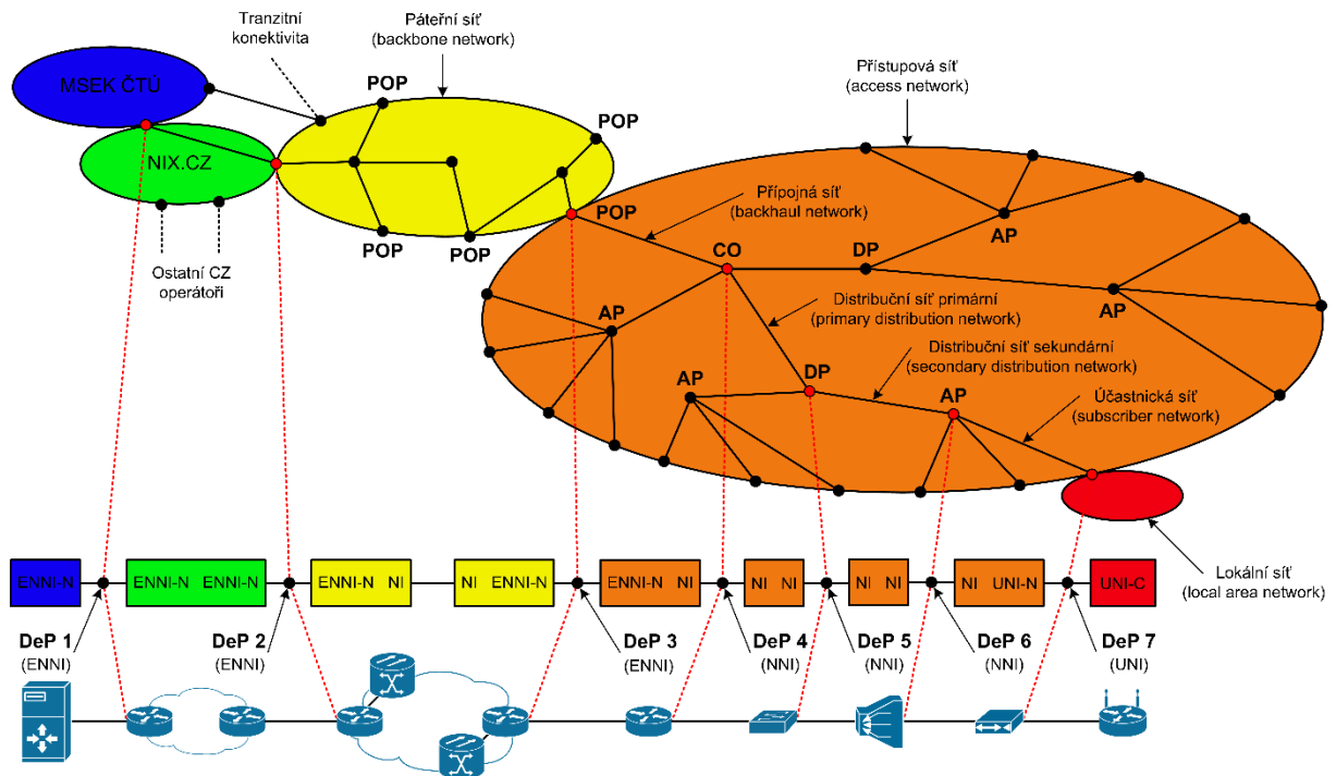
Obr. 5: Definované pozice demarkačních bodů (DeP) v rámci obecného schéma struktury přístupové sítě a jejího připojení do internetu
